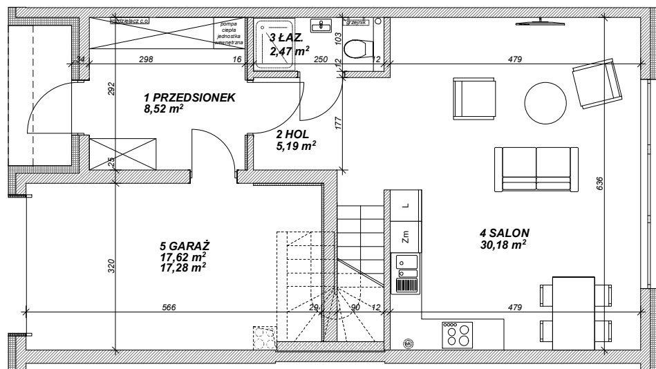
RZUT PARTERU
