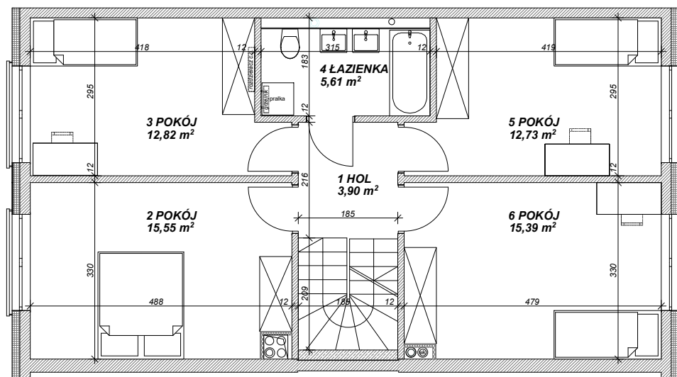
RZUT PIĘTRA
