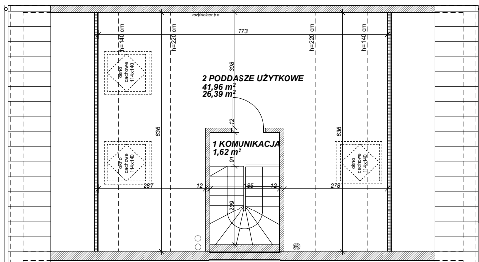
RZUT PODDASZA
