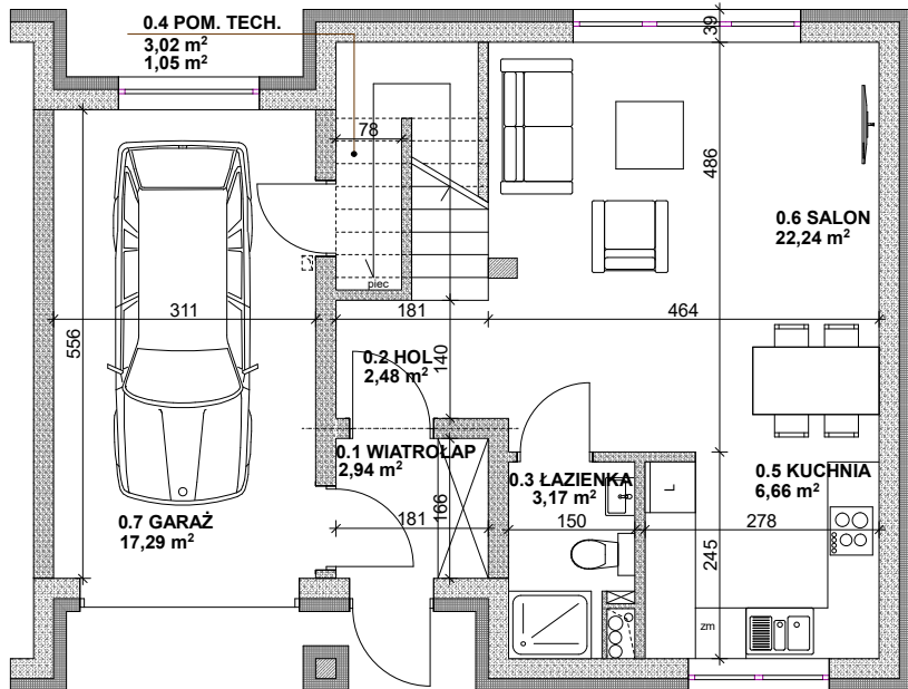
RZUT PARTERU
