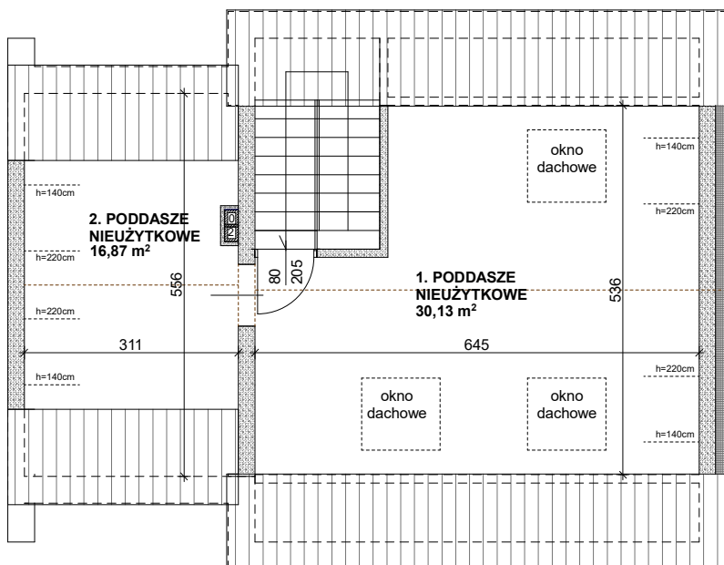
RZUT PODDASZA
