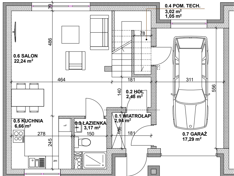
RZUT PARTERU
