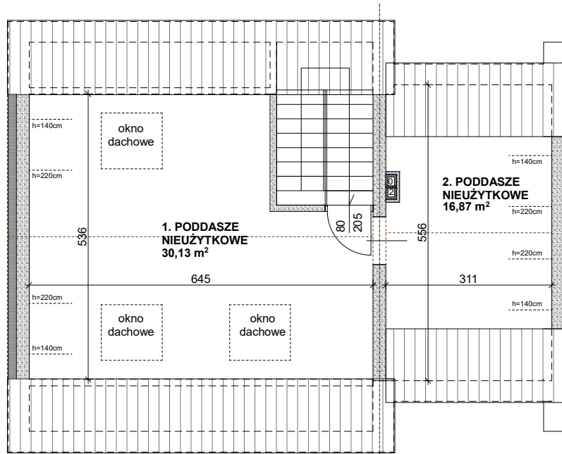
RZUT PODDASZA
