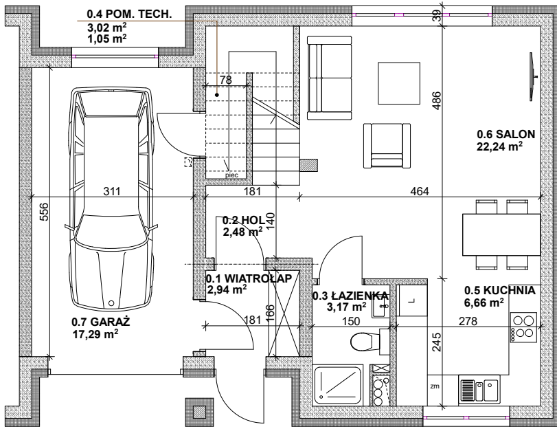
RZUT PARTERU
