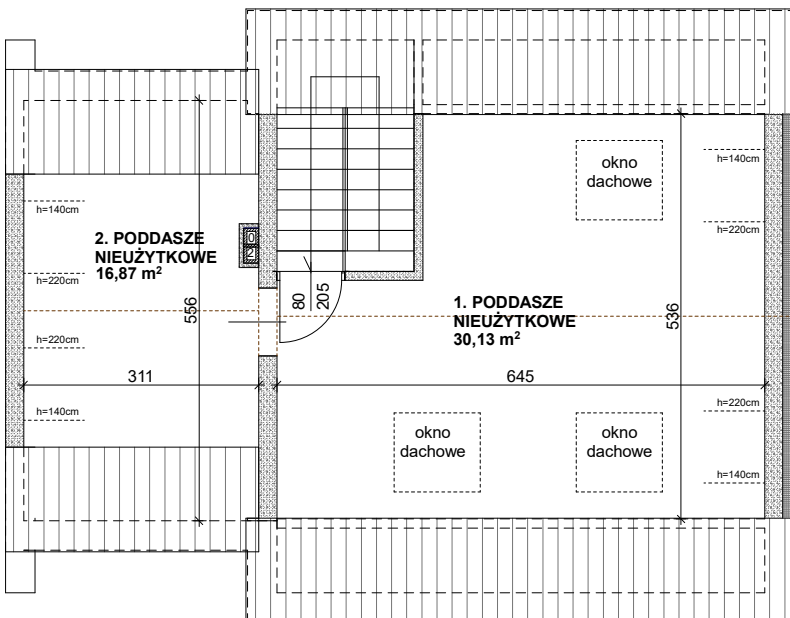
RZUT PODDASZA
