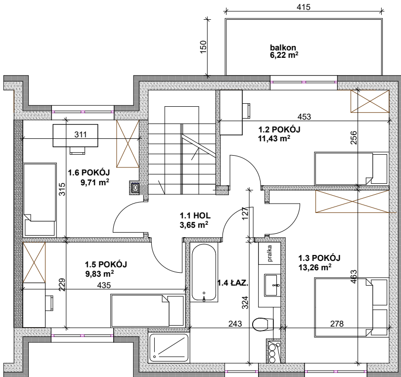
RZUT PIĘTRA
