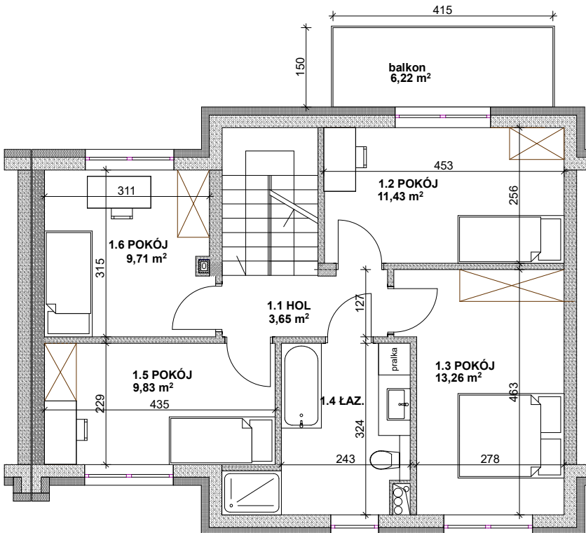
RZUT PIĘTRA
