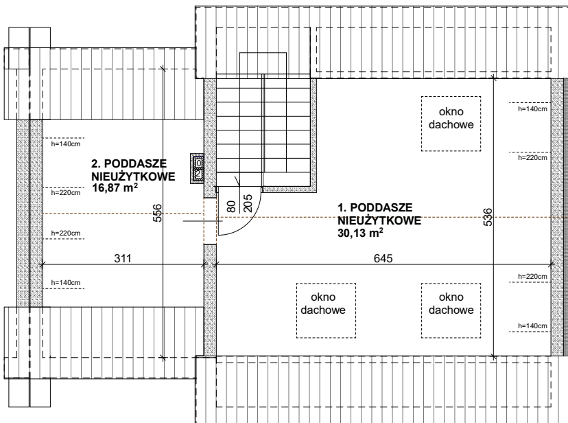
RZUT PODDASZA
