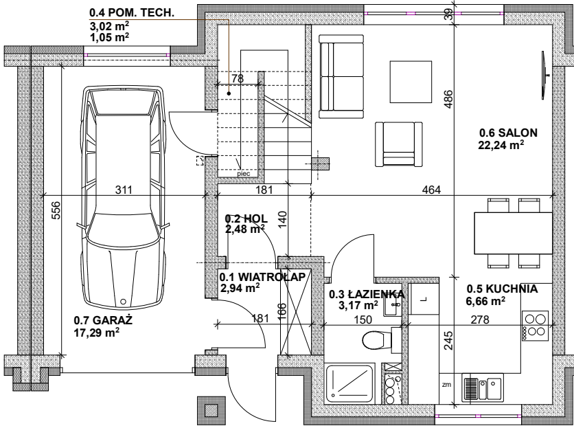
RZUT PARTERU
